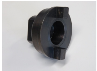
DL-M24L (CR 31098) Муфта удлинённая на 24 мм для ТНВД DENSO HP0
